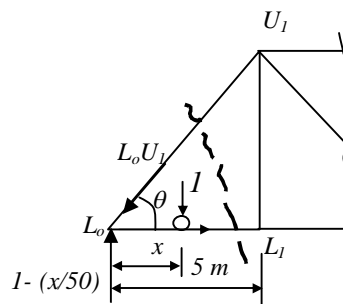
Fig. E2. Free body diagram
