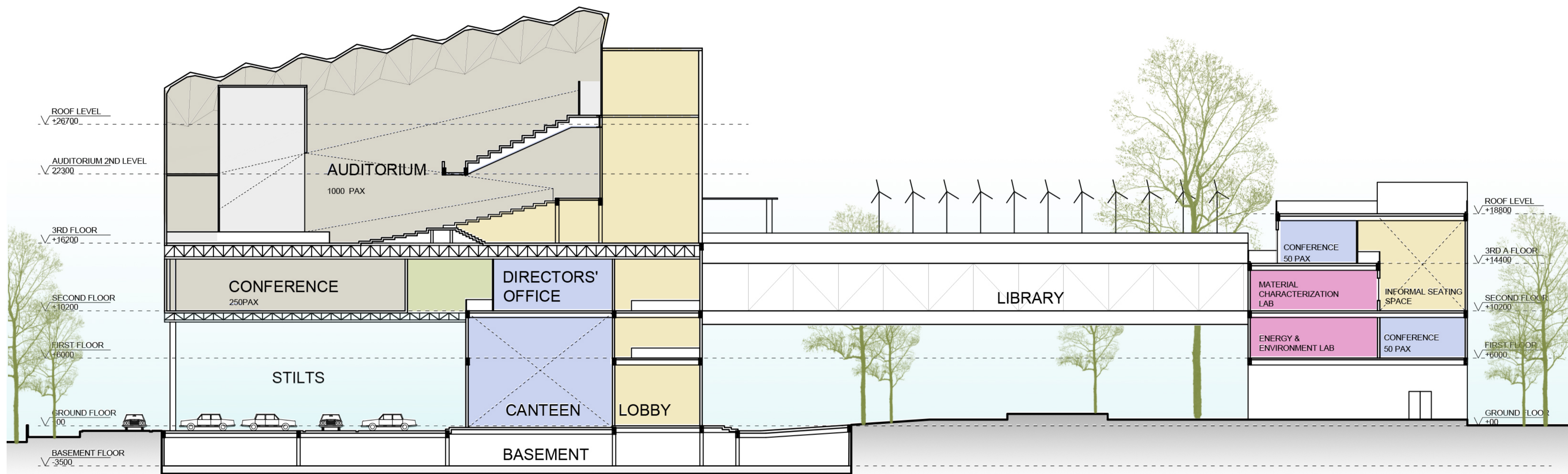
SECTION A-A' Scale - 1:200
